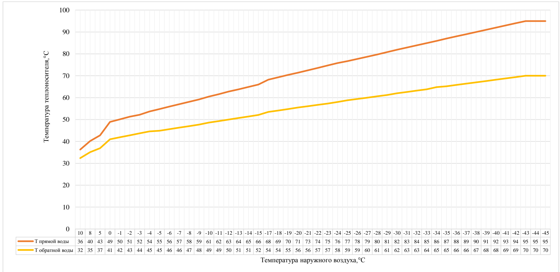
Рисунок 6 – Температурный график, зависимость температуры теплоносителя, отпускаемого с источника от температуры окружающего воздуха
